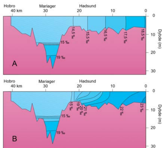
Figur 3.1 Længdeprofil af Mariager Fjord med angivelse af typisk saltholdighedsfordeling ved vindstille perioder (A) og efter periode med vestenvind (B). Fra Christensen (1997).
